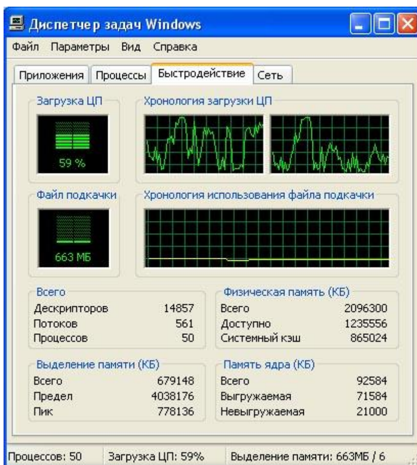
Рис. 19.2. Вкладка Быстродействие окна Диспетчер задач Window
