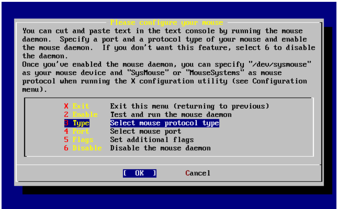
Рисунок 2-41. Выбор протокола мыши
